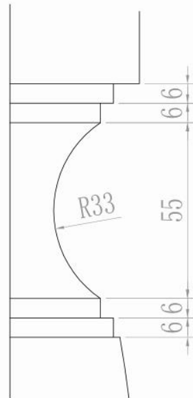
A—A放大图
