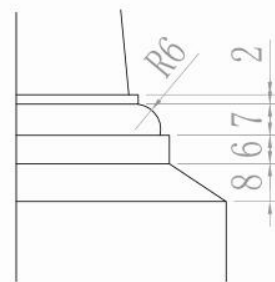
B—B放大图
